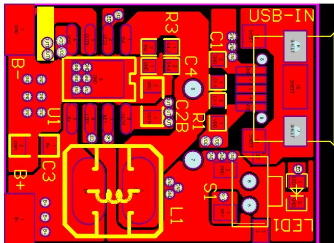
Fig1.顶层整体布局
